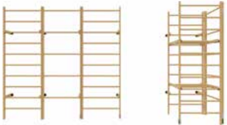
3-delig wandrektoren Hoogte: 2,90 meter 2x tussenraam + 2x 10 sporten + 1x 5 sporten
